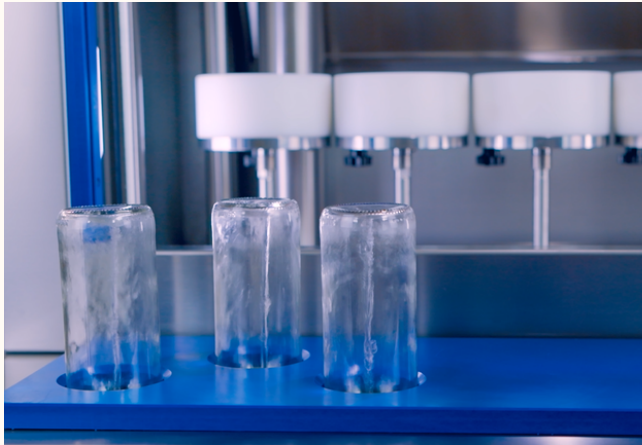
UNITÉ DE RINÇAGE À 6 POSTES
